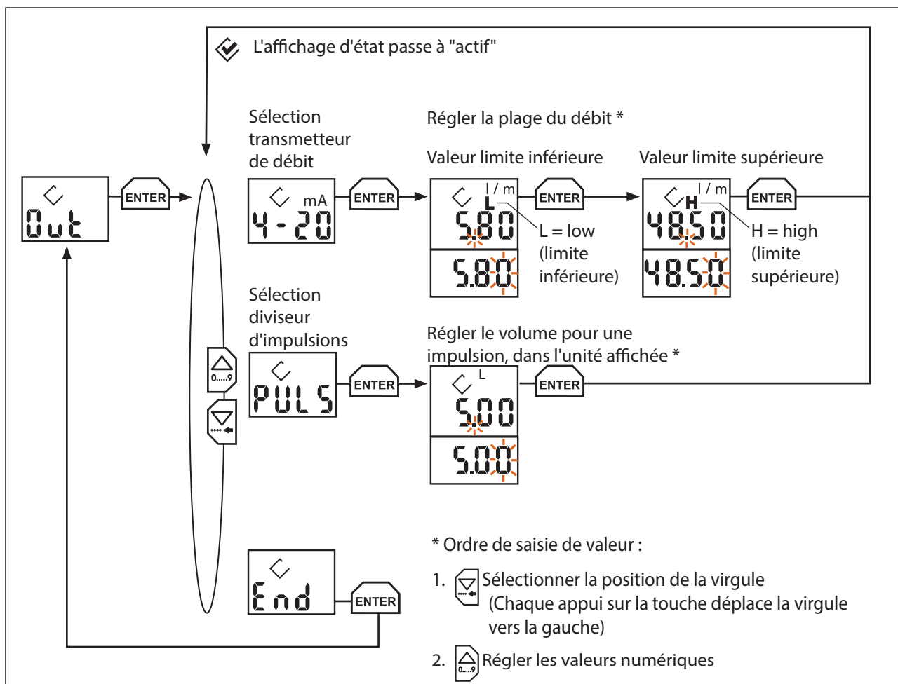
Fig. 17 : Out – Régler de la sortie ; fonctionnement en tant que transmetteur de débit ou diviseur d'impulsions
