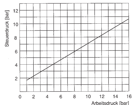
Steuerdruckdiagramm für Bestell-Nr. 031 582
