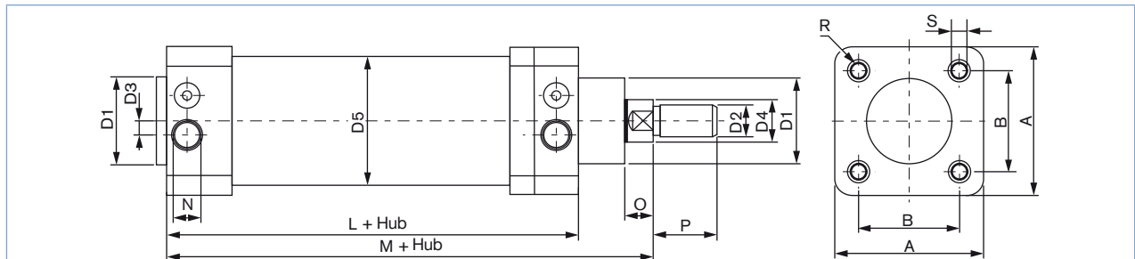
Zylinder mit Kolbendurchmesser 32 ... 50 mm nach ISO 6431
