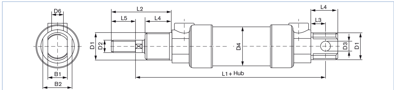
Zylinder mit Kolbendurchmesser 12 ... 25 nach ISO 6432 (CETOP) Rp 52 P
