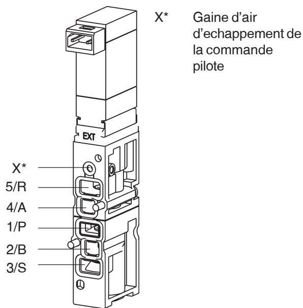
Fig.: Raccordement fluide (Vanne - Type 6525)
