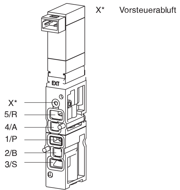
Bild: Fluidischer Anschluss (Ventil - Typ 6525)
